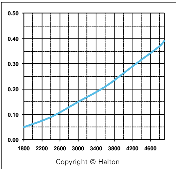
KVO - 6 Filters per side
