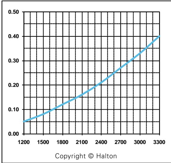
KVO - 5 Filters per side
