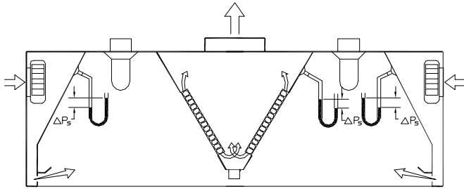
KVW/KVO/KVR - 2 Filters Per Side
