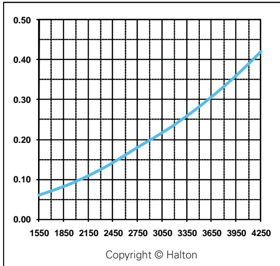
KVV/KVO/KVR - 6 Filters Per Side
