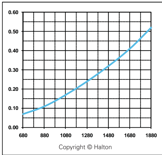
KVW/KVO/KVR - 2 Filters Per Side
