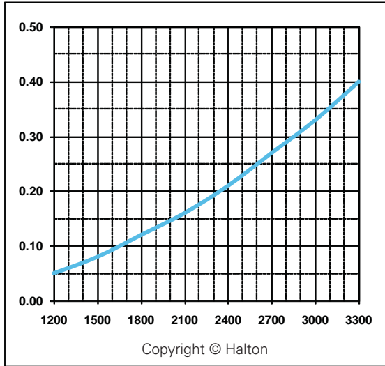
KVV/KVO/KVR - 5 Filters Per Side
