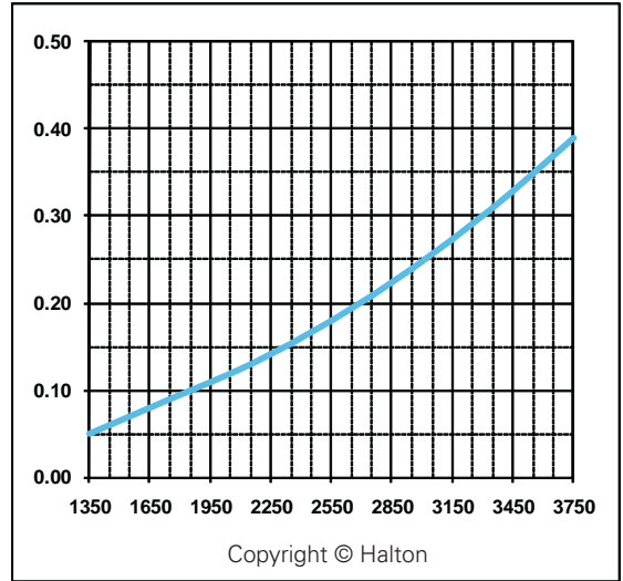
KVV/KVO/KVR - 5.5 Filters Per Side
